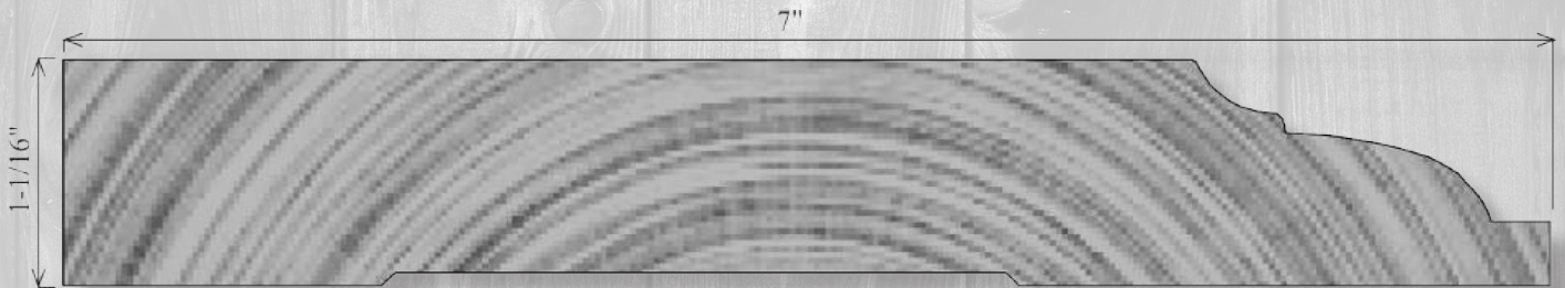
B700 1-1/16" x 7"
